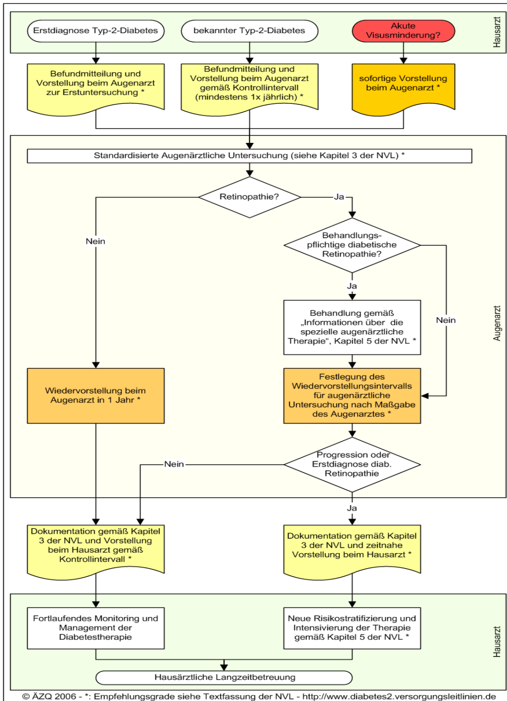
Abbildung 2: Flussdiagramm Patientenmanagement
