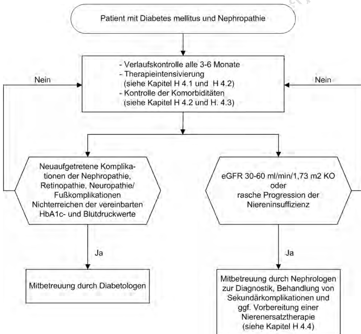
Algorithmus 3: Schnittstellendefinition
